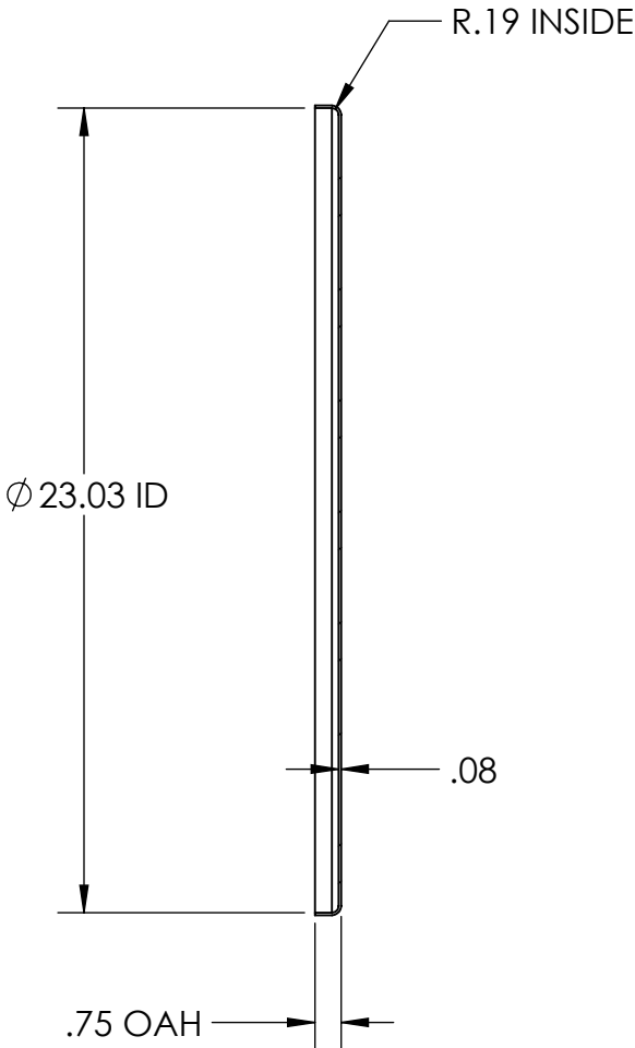
SECTION A-A SCALE 1 : 6
